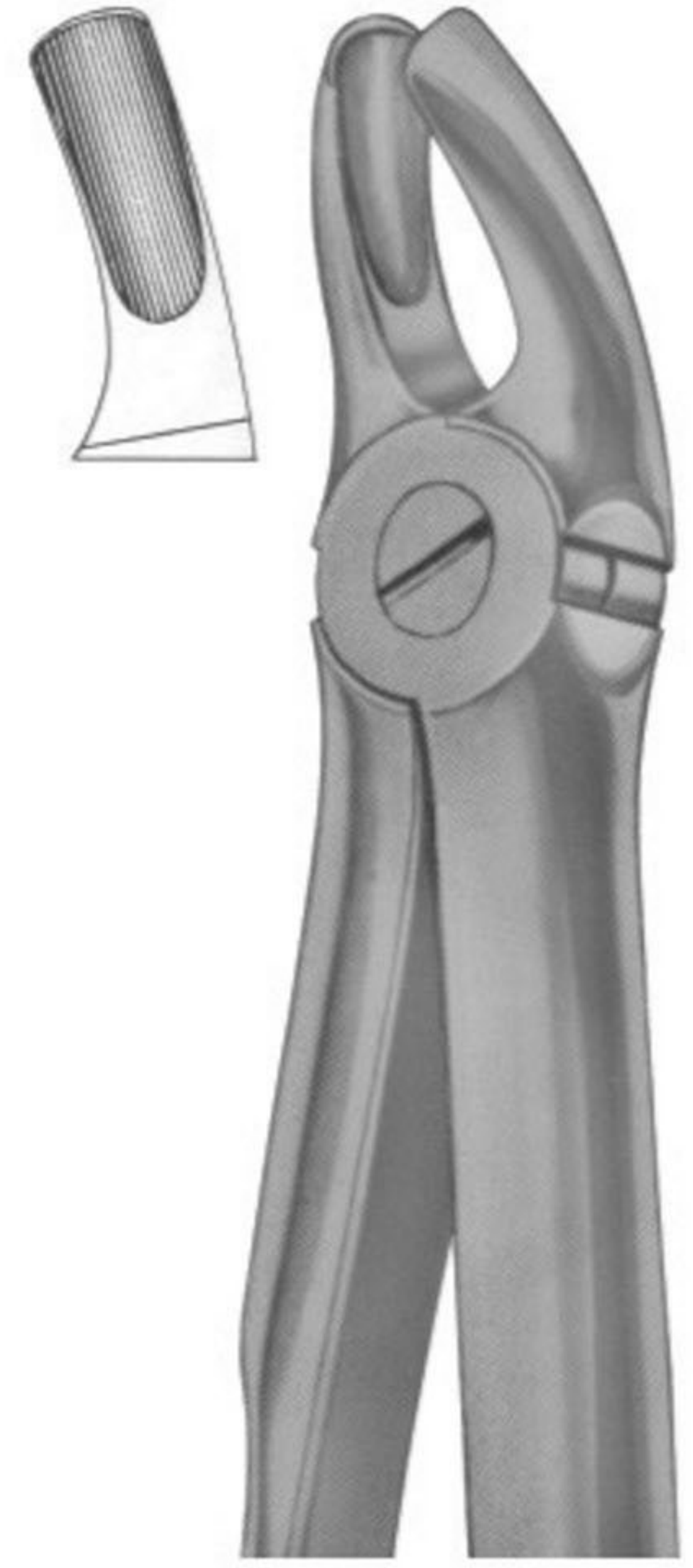
1155 Fig. 18B upper molars
