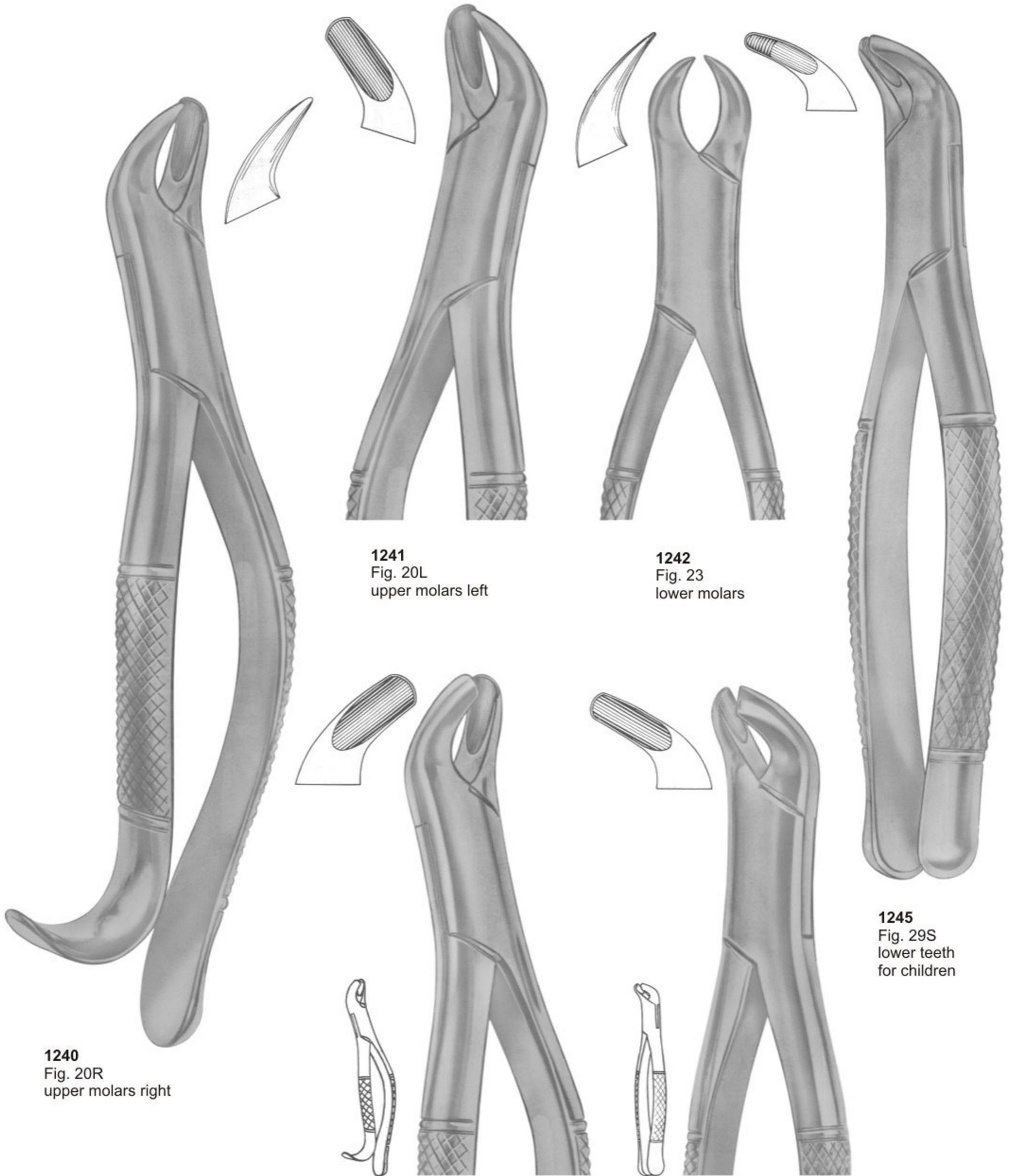
1243 Fig. 24 upper molars
